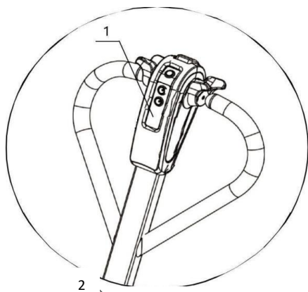
Рис.6 - Функциональные кнопки на рукояти
